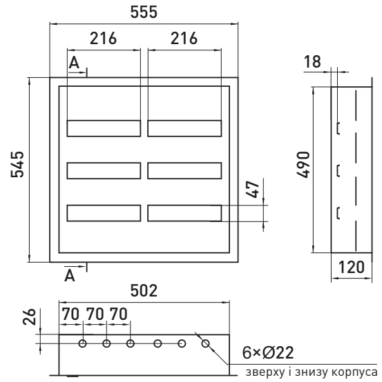
e.mbox.pro.w.72z IP31
