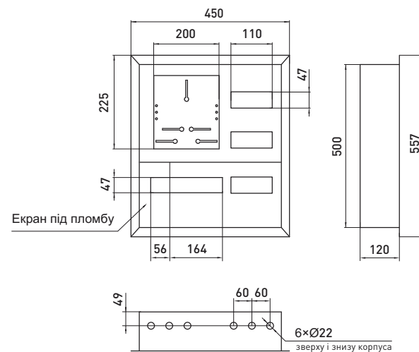
e.mbox.pro.w.f3.27z IP31
