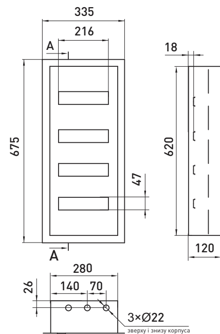
e.mbox.pro.w.48z IP31
