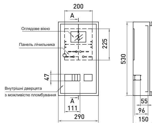
e.mbox.pro.n.f3.9z IP54
