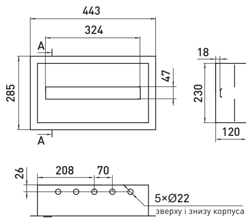
e.mbox.pro.w.18z IP31
