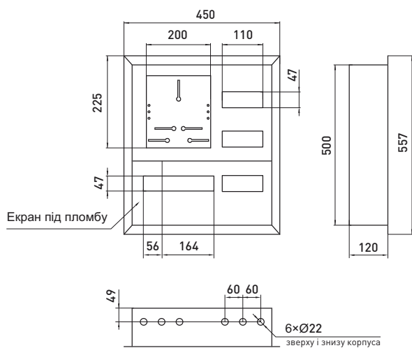
e.mbox.pro.w.f3.12z IP31
