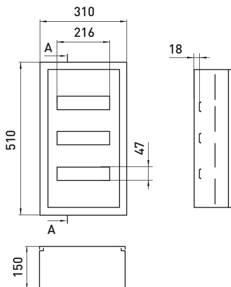
e.mbox.pro.n.36z IP54
