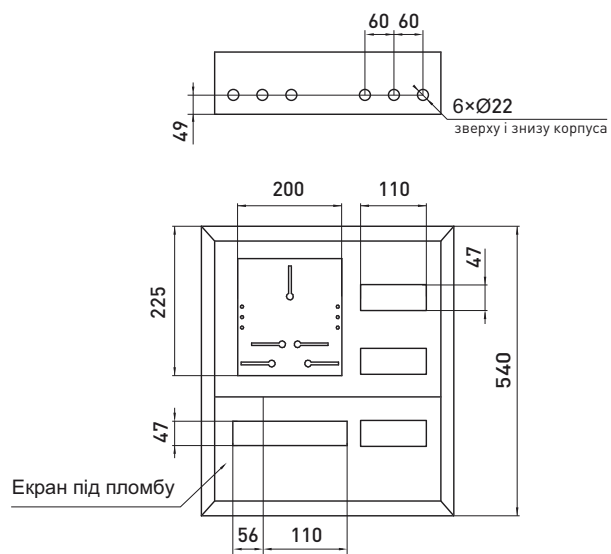
e.mbox.pro.n.f3.27z IP31
