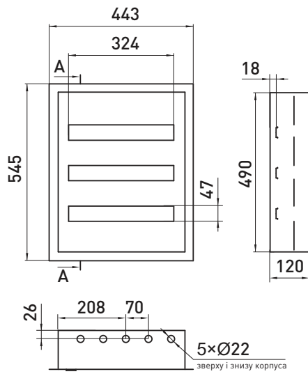
e.mbox.pro.w.54z IP31
