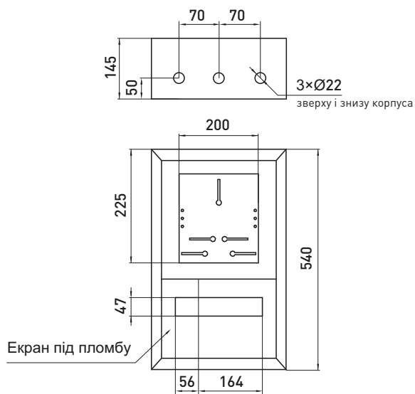
e.mbox.pro.n.f3.12z IP31
