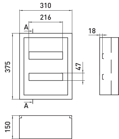
e.mbox.pro.n.24z IP54
