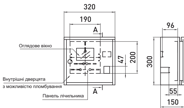
e.mbox.pro.n.f1.4z IP54
