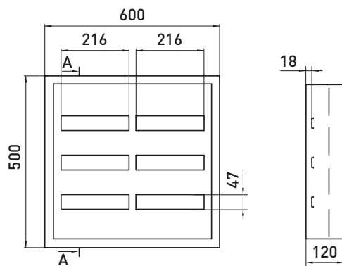
e.mbox.pro.n.72z IP31
