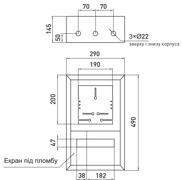
e.mbox.pro.n.f1.12z IP31
