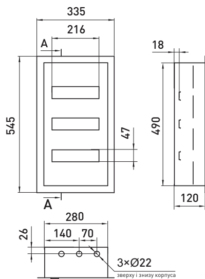
e.mbox.pro.w.36z IP31
