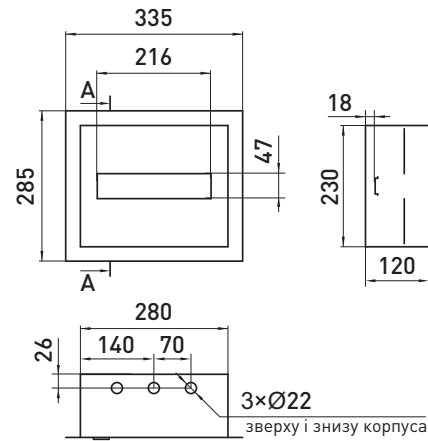
e.mbox.pro.w.12z IP31
