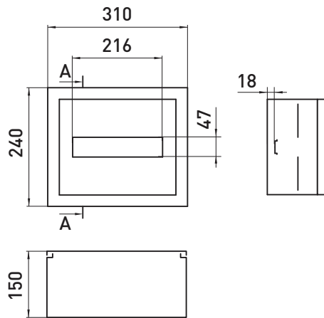
e.mbox.pro.n.12z IP54
